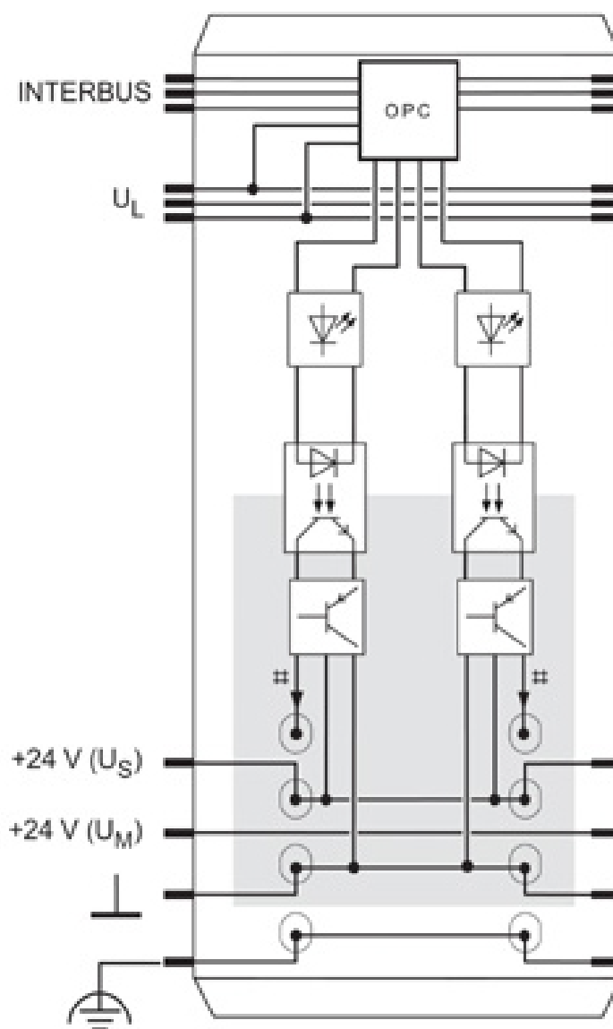
blokschema
