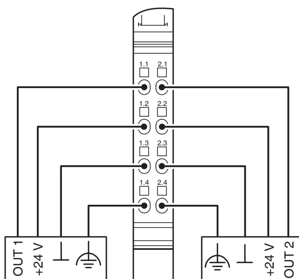
aansluitschema
