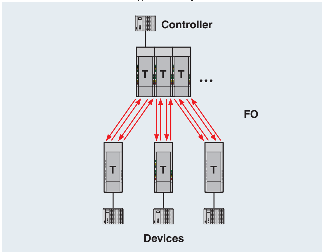
Redundante sterstructuur
