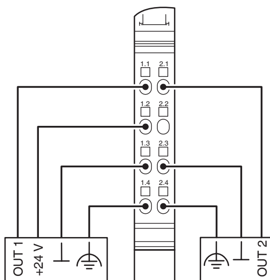
aansluitschema
