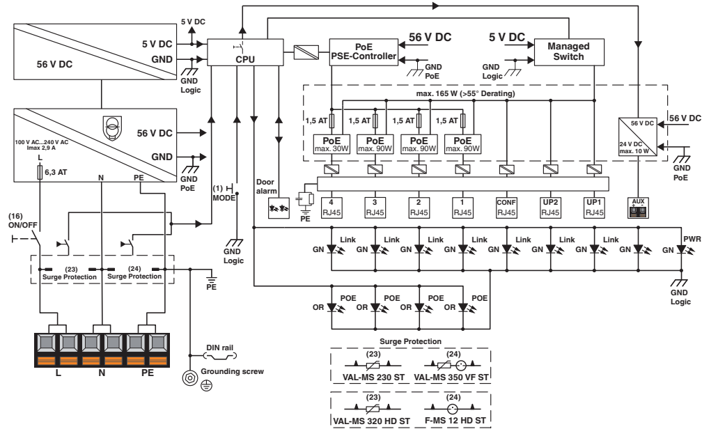
schakelschema
