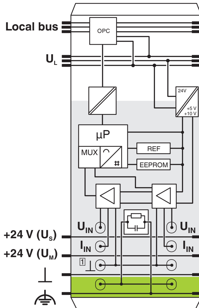
blokschema
