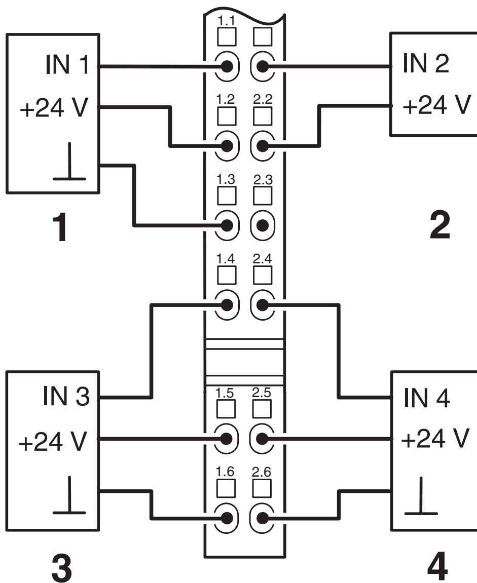
aansluitschema
