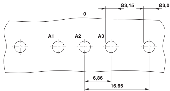
boorsjabloon/soldeerpadgeometrie
