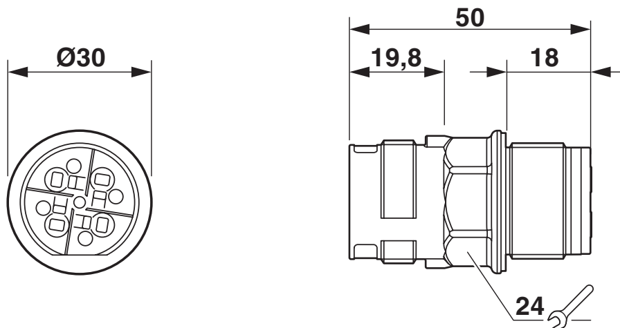
Maatschets
