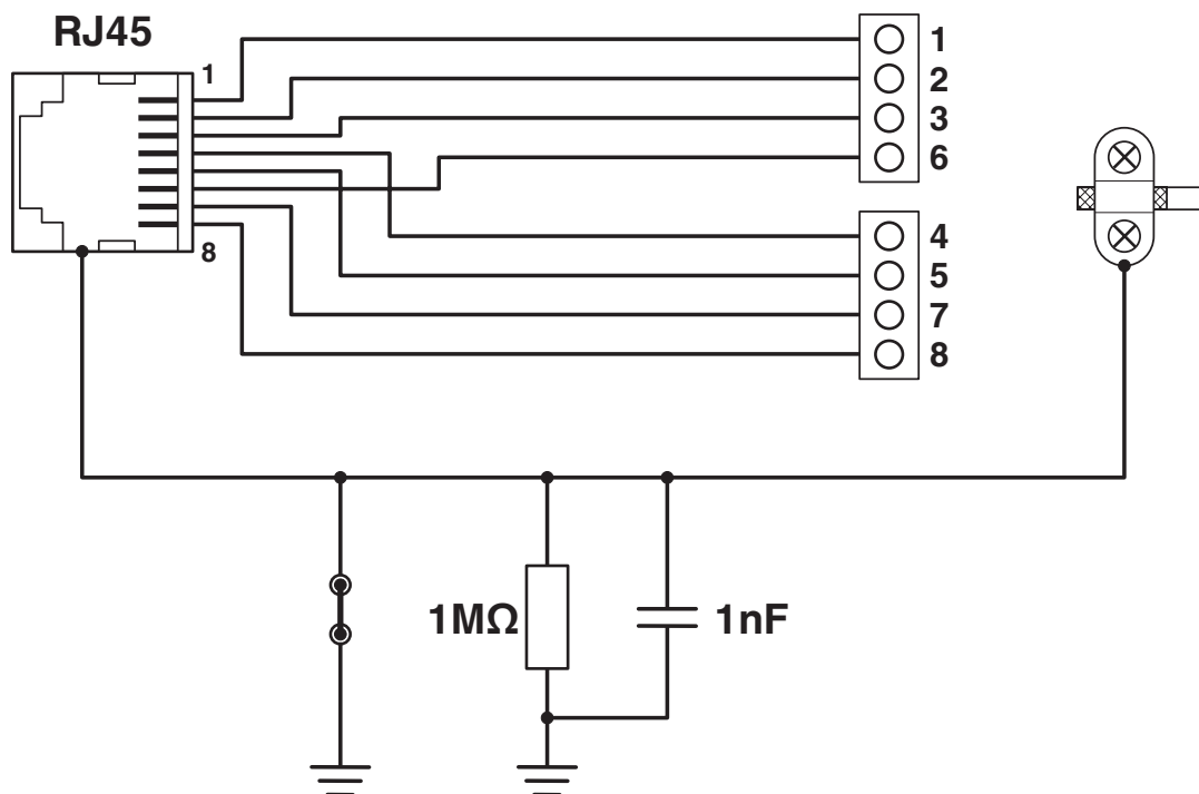
schakelschema
