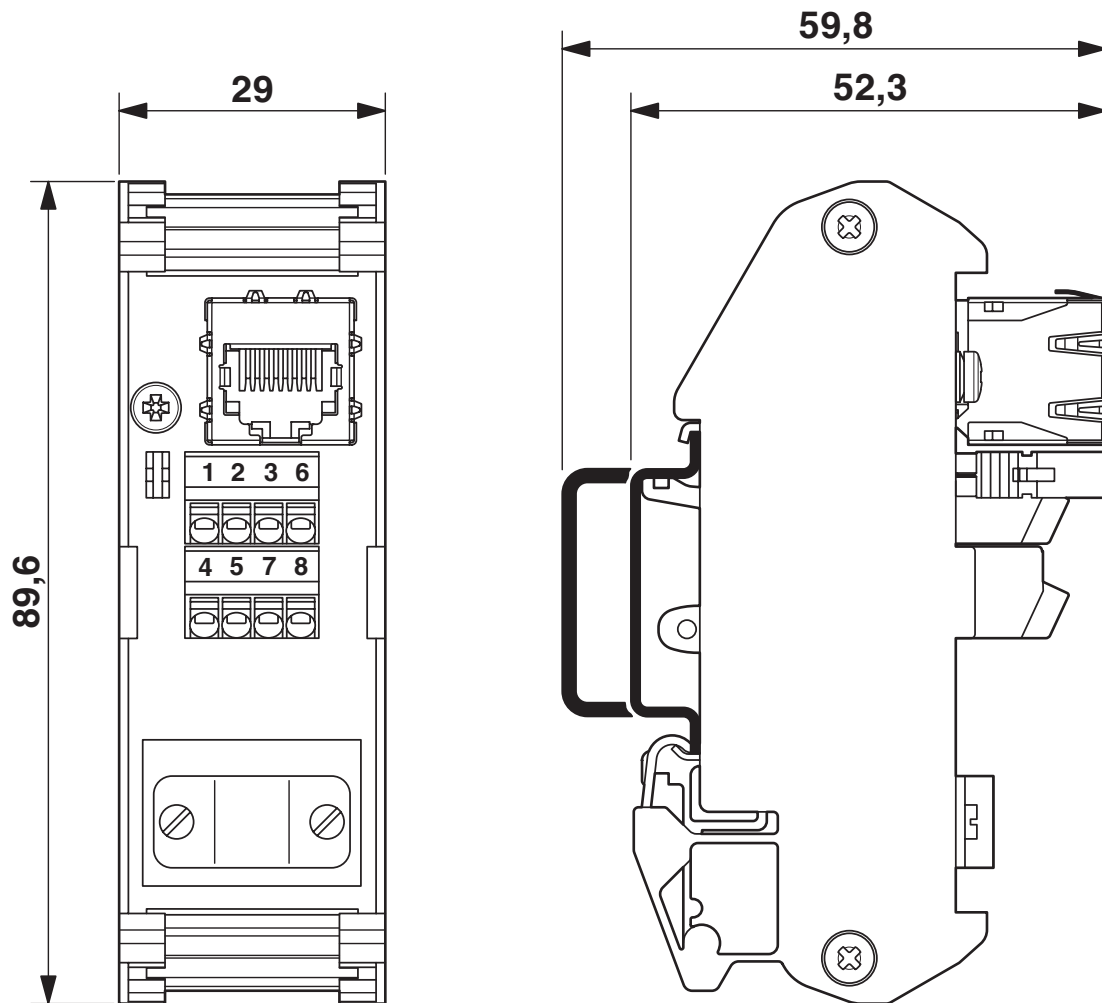
Maatschets
