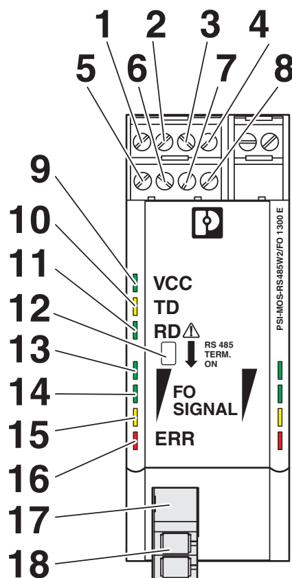
schematekening
