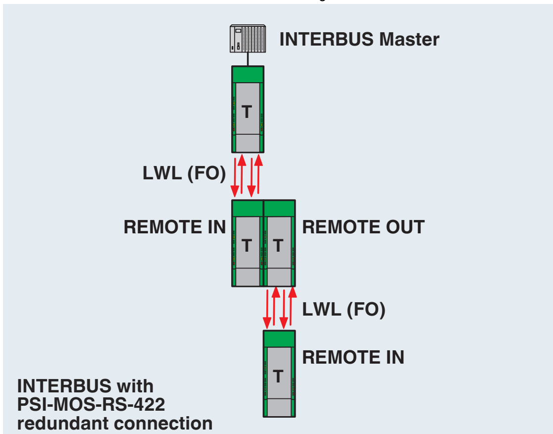
functietekening
