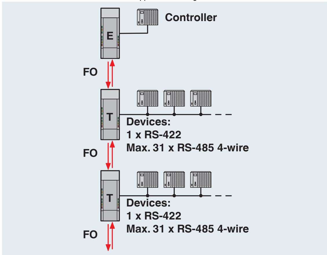
Controller-device-lijnstructuur
