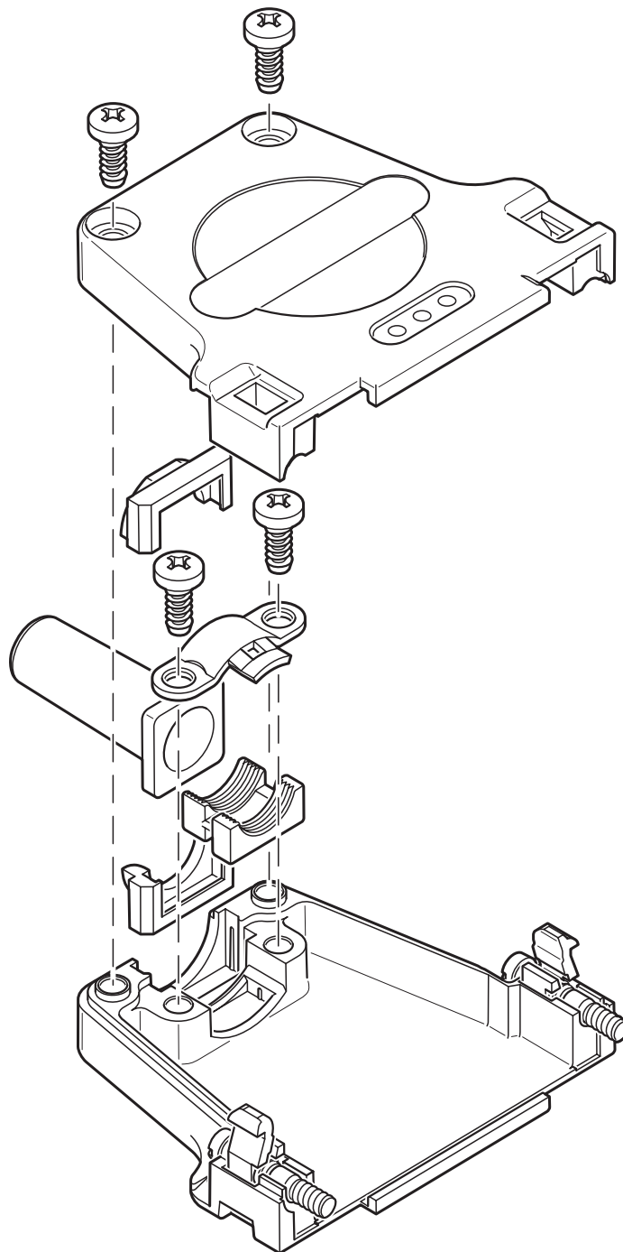
schematekening
