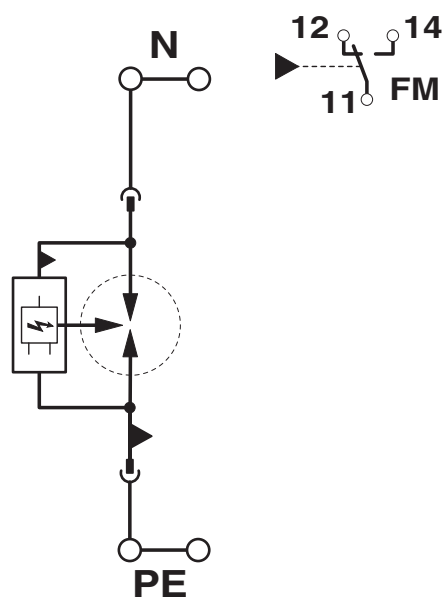
schakelschema
