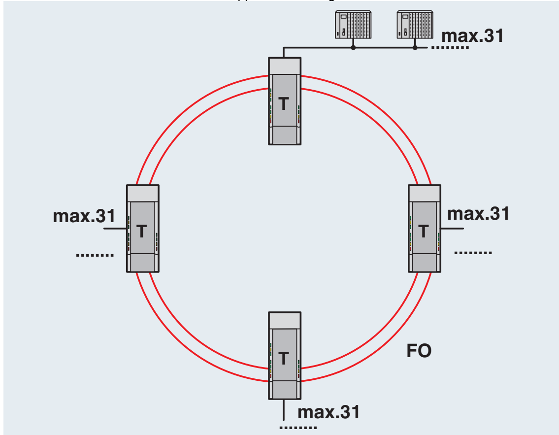
Redundante glasvezelring
