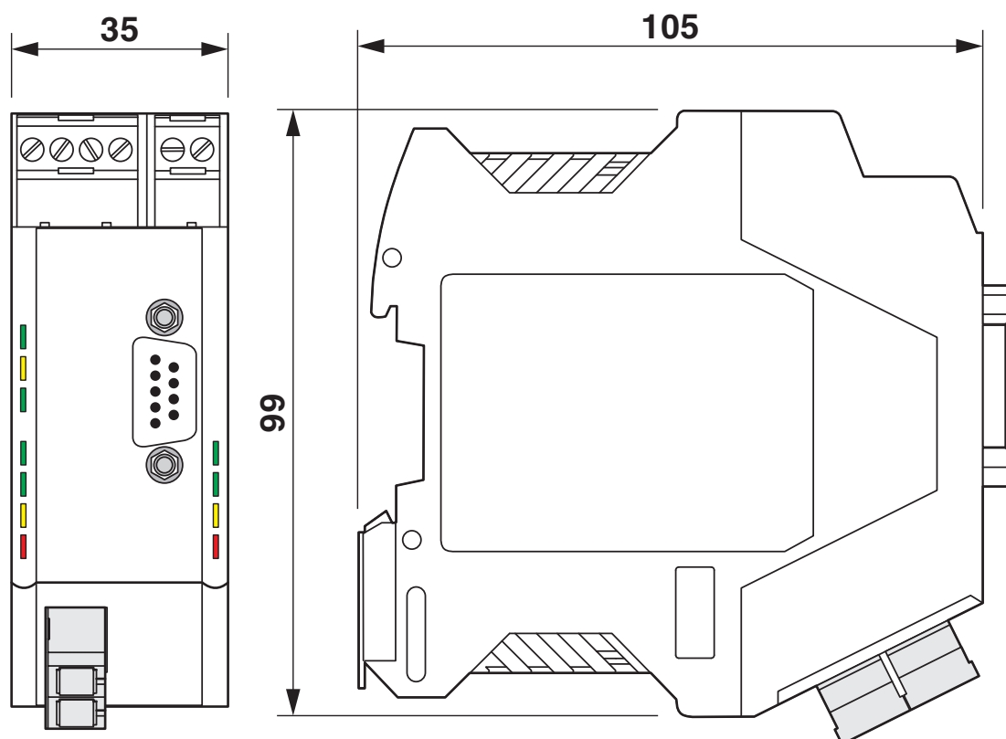
Behuizingsafmetingen
