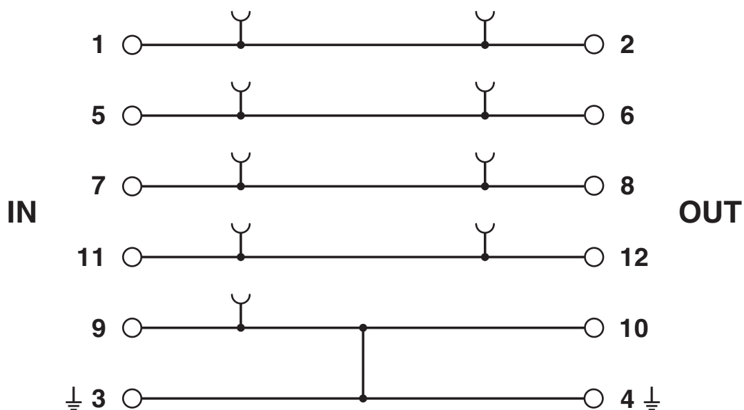
schakelschema
