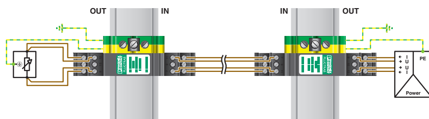
applicatietekening
