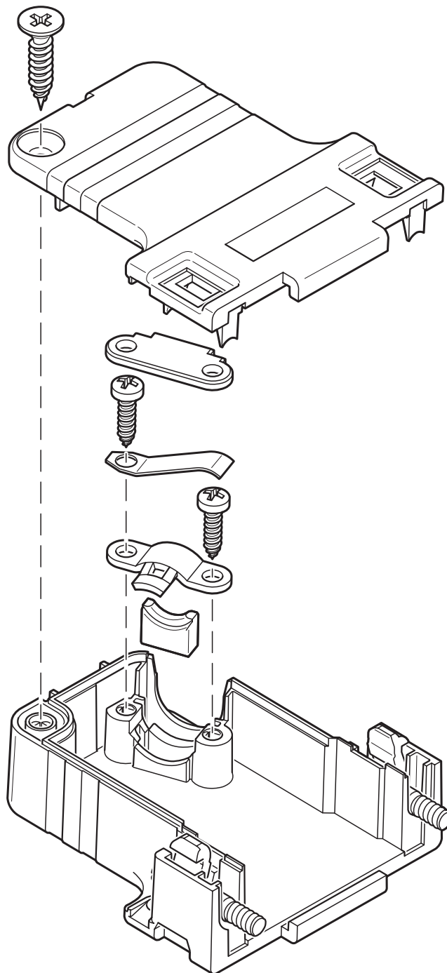
schematekening
