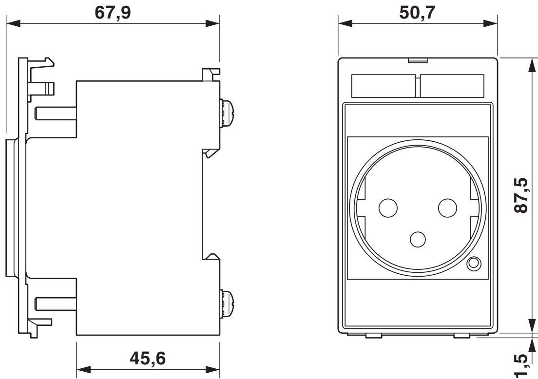
Wandcontactdoosinzet
