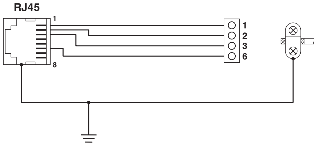
schakelschema
