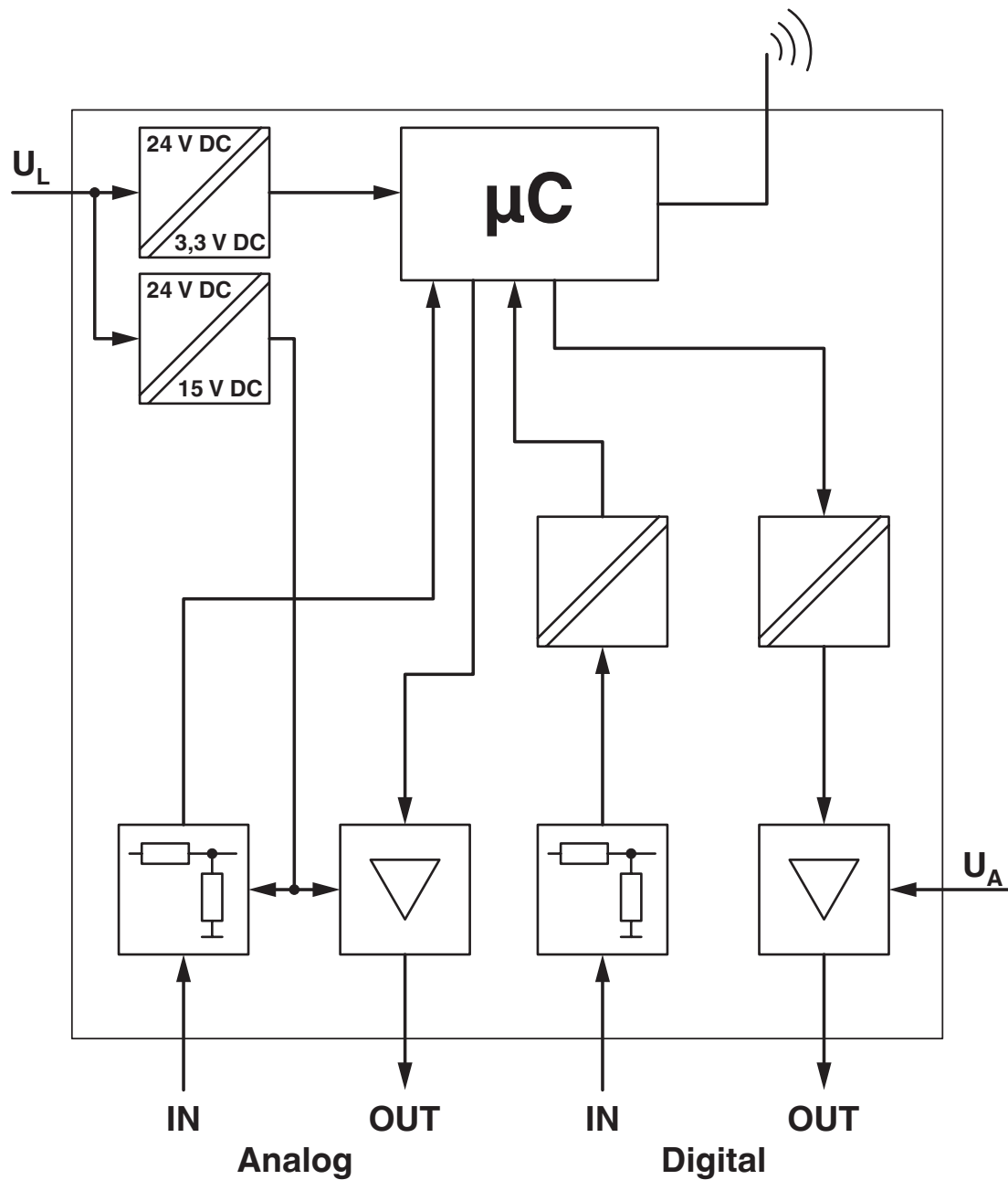
blokschema
