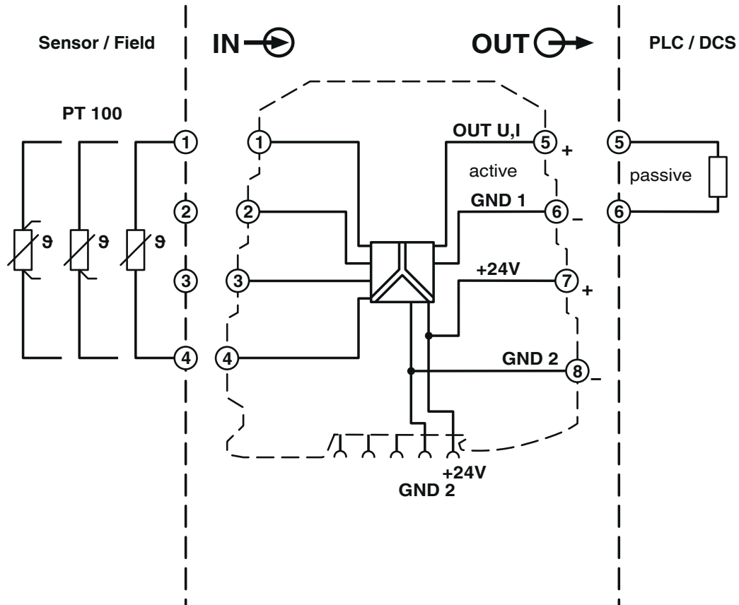
blokschema
