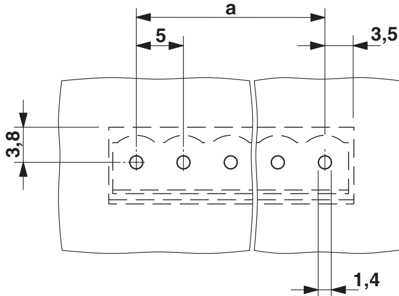
boorsjabloon/soldeerpadgeometrie
