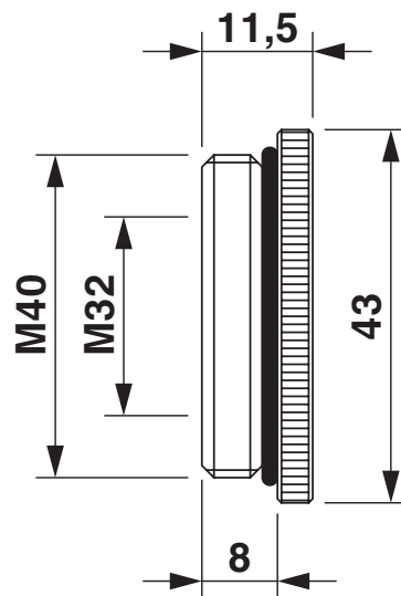
Maatschets
