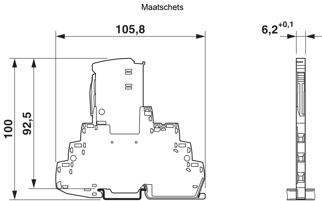
schematekening
