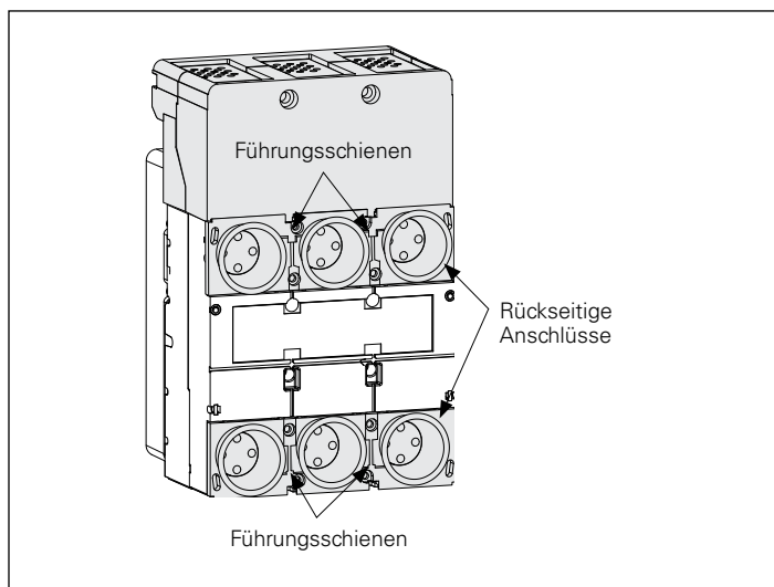
Abbildung 5. Festeinbauswitcher mit rückseitigen Anschlüssen (Rückansicht)
