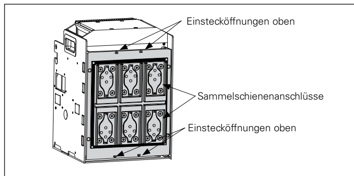
Abbildung 1. Kasette (Rückansicht)
