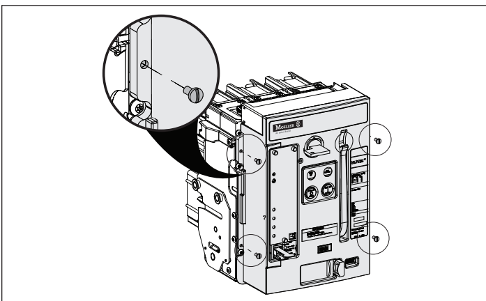
Abbildung 4 - Schritt 1
