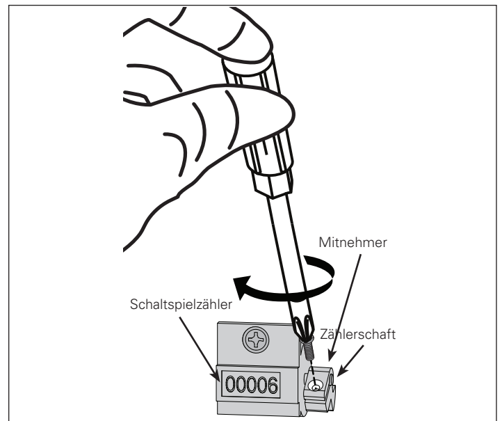
Abbildung 6 - Schritt 3
