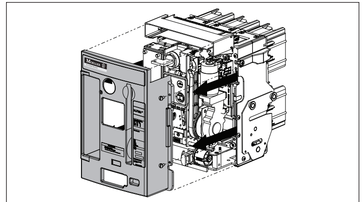
Abbildung 5 - Schritt 2
