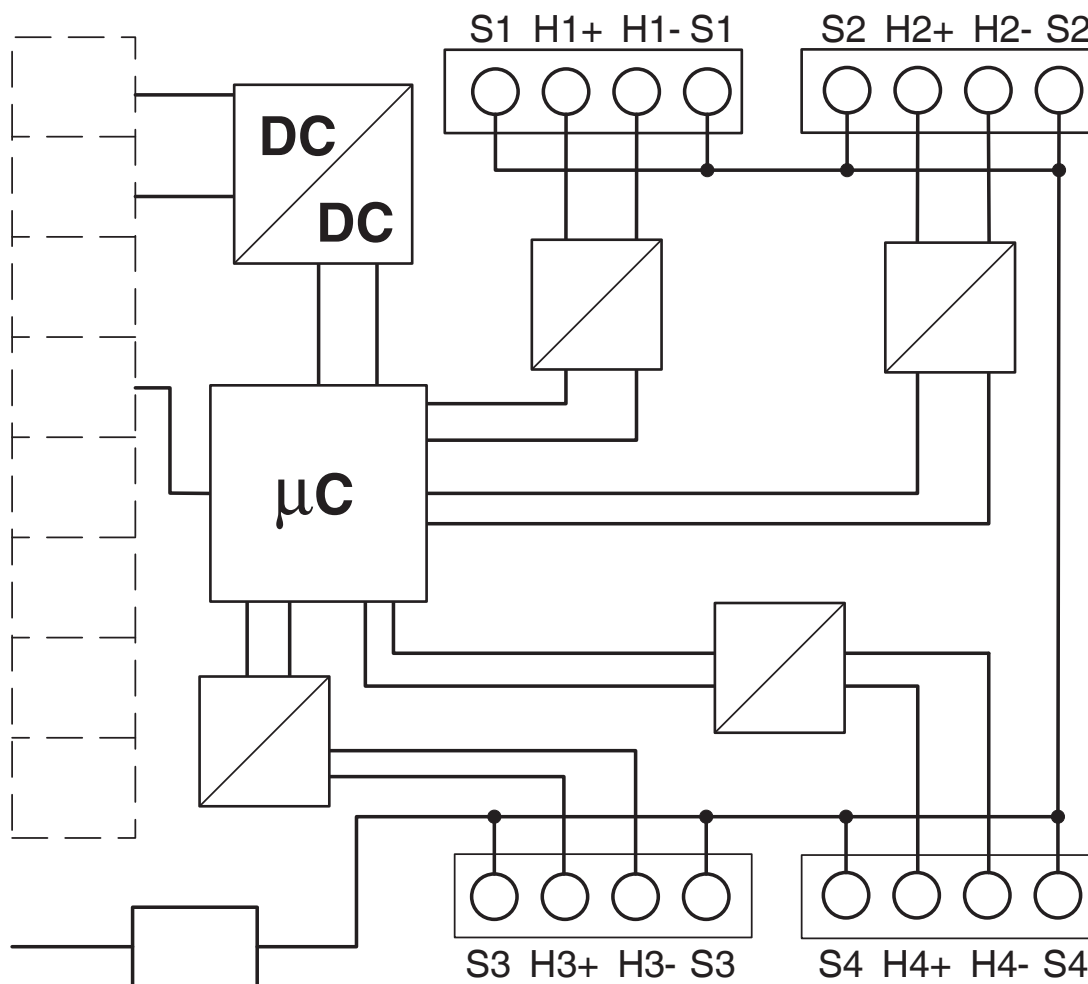
blokschema
