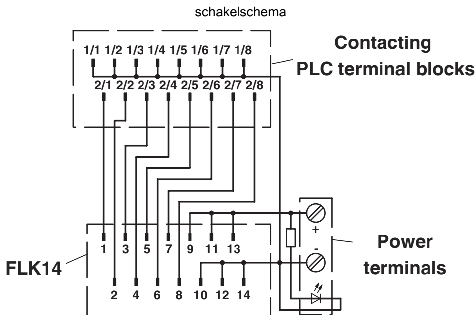
Aansluitschema PLC-V8/FLK14/IN/M
