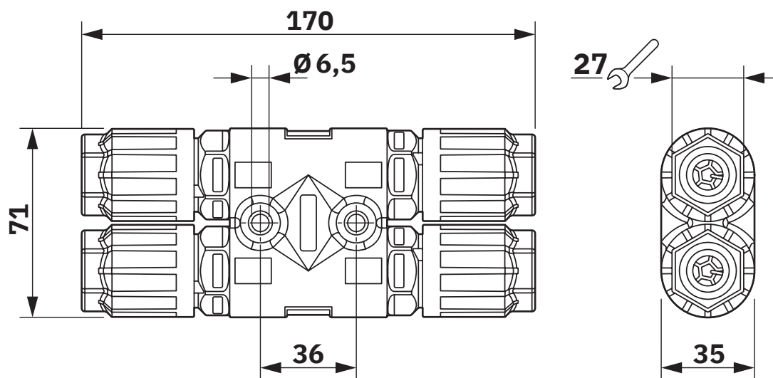
Maatschets
