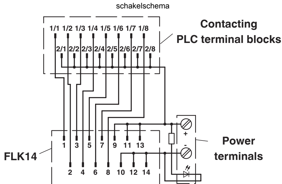
Aansluitschema PLC-V8/FLK14/IN
