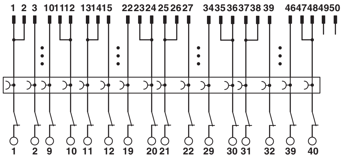
Aansluitschema FLKM 50/KDS3-MT/PPA/S7-300
