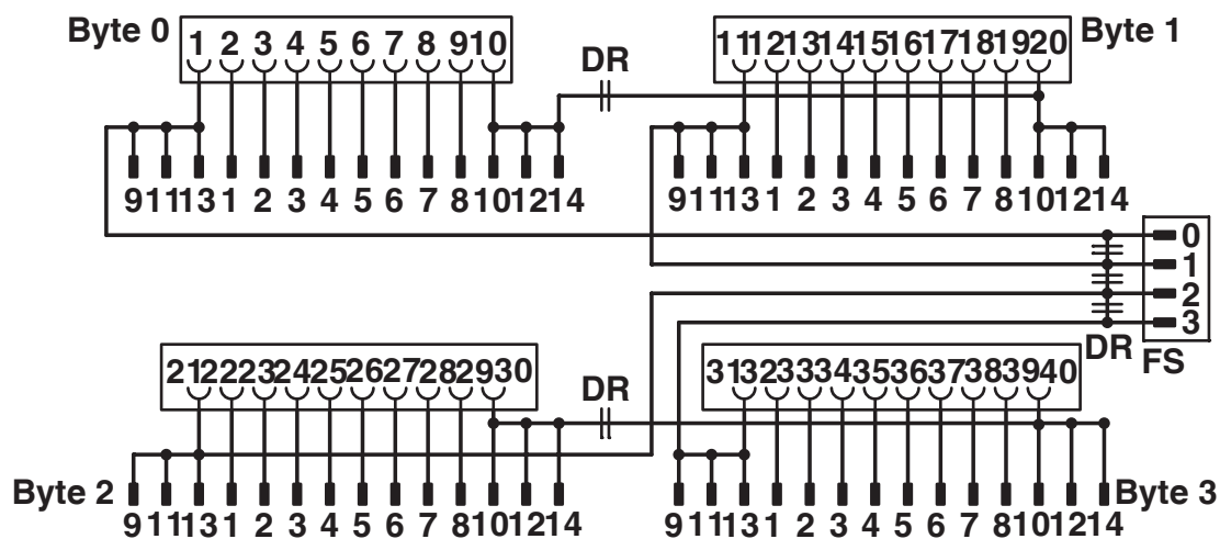
Aansluitschema FLKM 50/4-FLK14/PA-S300
