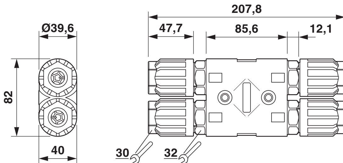
Maatschets
