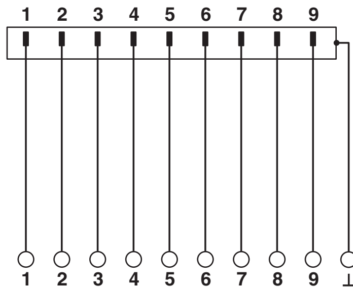
schakelschema
