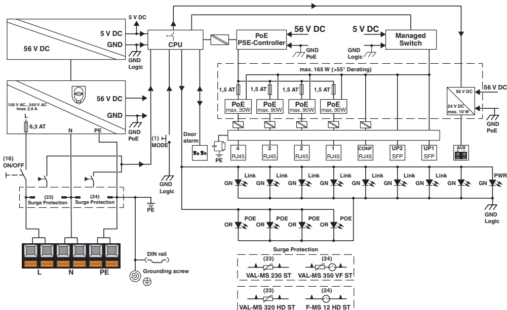
schakelschema
