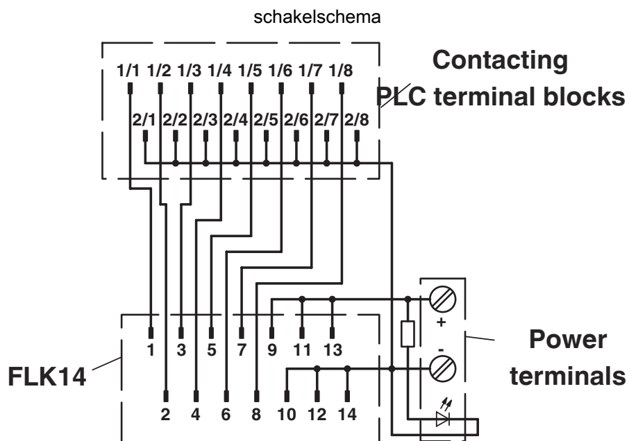
Aansluitschema PLC-V8L/FLK14/OUT
