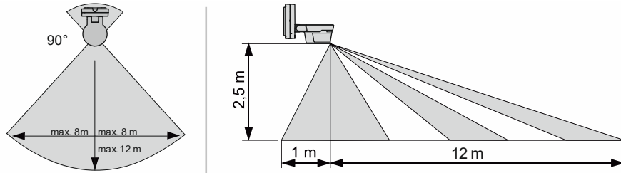
Abb. 4: Erfassungsbereich 6851/9-xxx
