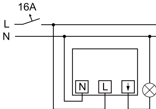
Abb. 7: Standardanschluss
