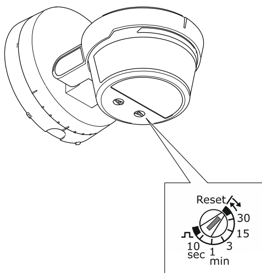
Abb. 41: Wahlschalter Reset
