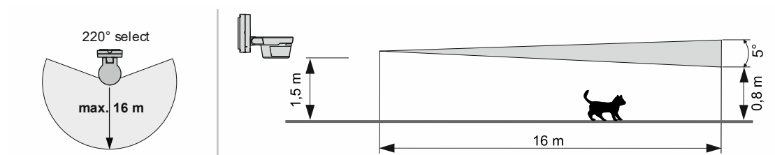
Abb. 6: Erfassungsbereich 6851/22S-xxx
