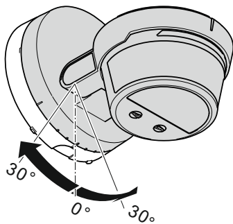
Abb. 35: Erfassungsbereich an Hanglage anpassen
