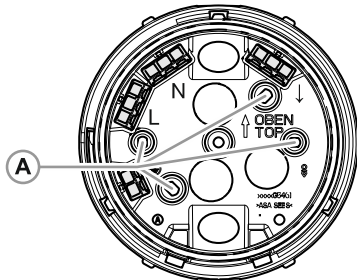
Abb. 13: Anschraubmöglichkeiten Sockel
