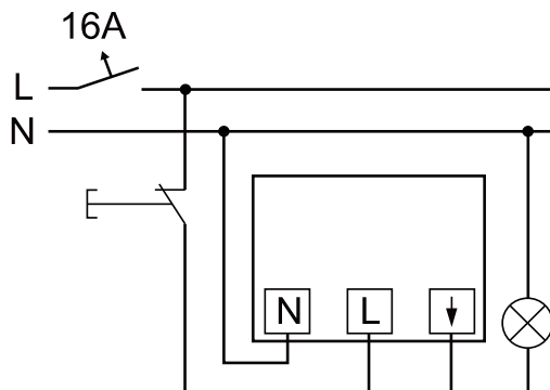
Abb. 8: Standardanschluss mit Öffnertaster
